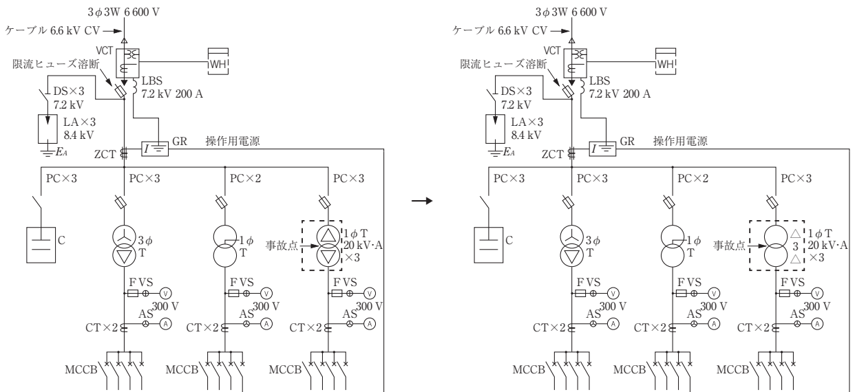
◎3 か月目レポート自由提出課題(T4) 図1 単線結線図(変圧器の過負荷焼損) 誤) 正)
